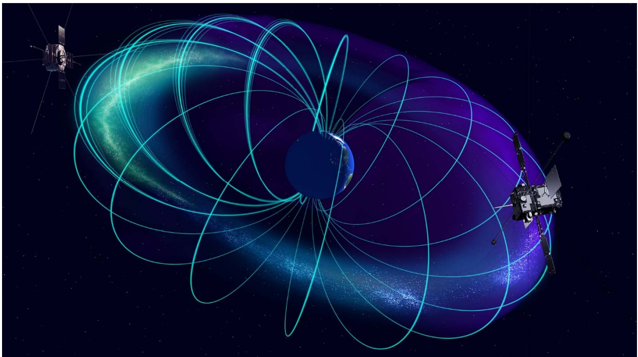
図1：ヴァン・アレン帯の電子が加速される場所をあらせ衛星と Van Allen Probes 衛星で特定
